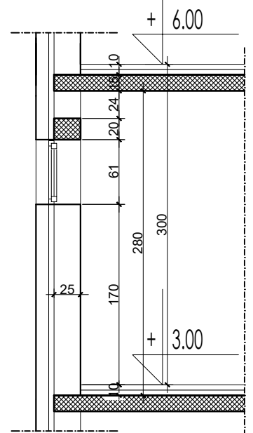
Пресек - спрат
