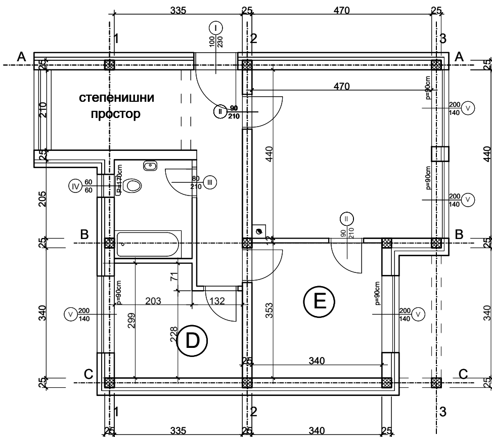
Скица основе спрата Р 1:100
