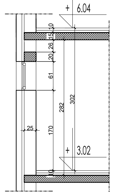
Пресек - спрат
