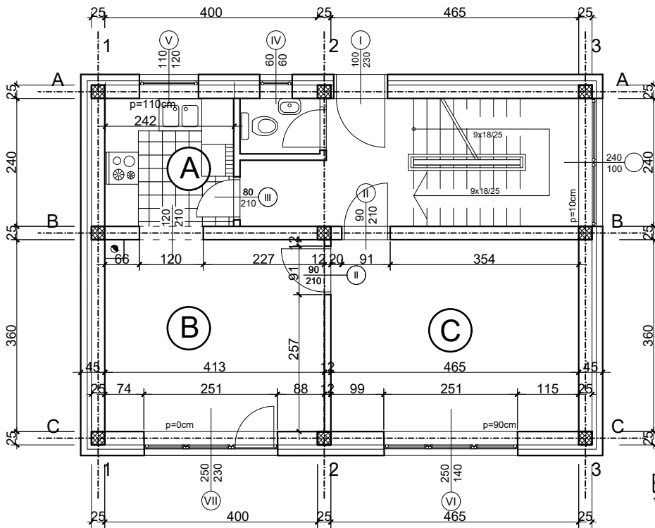
Скица основе приземља Р 1:100
