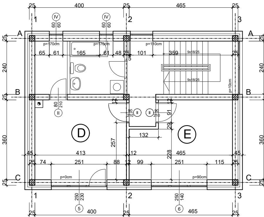
Скица основе спрата Р 1:100
