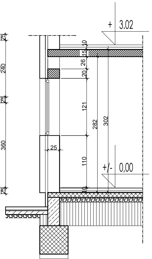
Пресек - приземље
