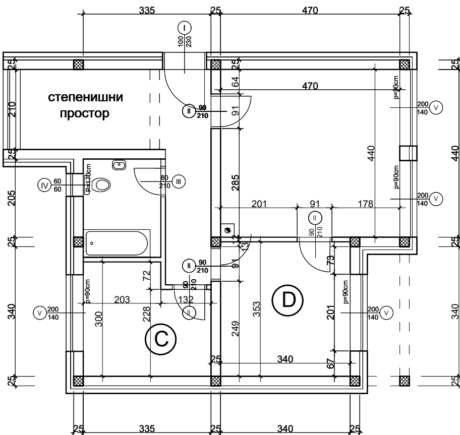
Скица основе спрата Р 1:100
