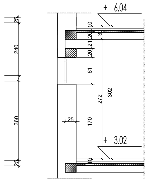
Пресек - спрат
