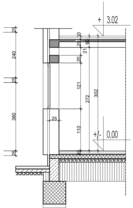
Пресек -приземље
