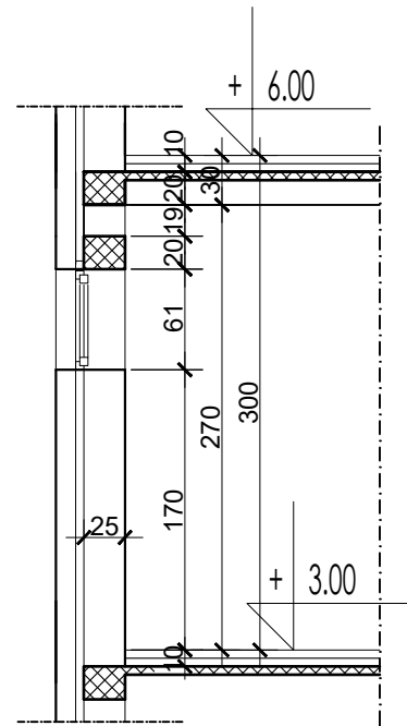
Пресек спрат купатило
