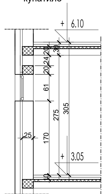
Пресек спрат купатило
