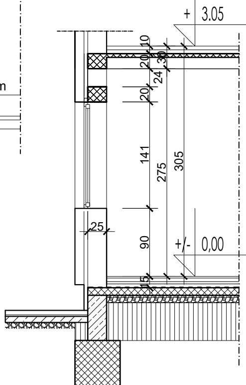
Пресек приземље кухиња и WC
